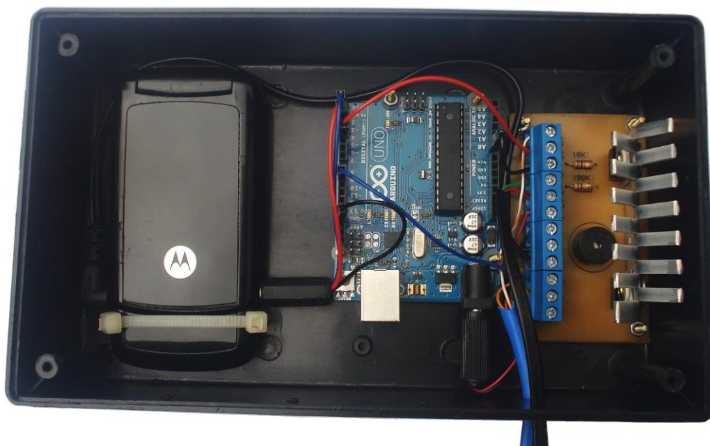
Figura 18: Ligação entre módulos e o celular
