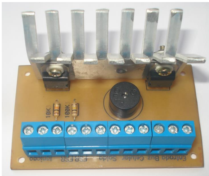
Figura 15: Módulo de integração com o Arduino finalizado
