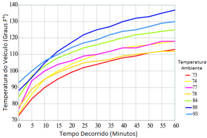
Figura 1: Aumento de temperatura versus temperatura ambiente
