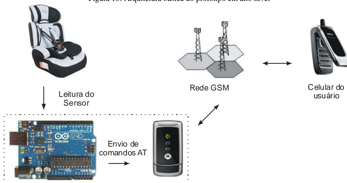
Figura 13: Arquitetura básica do protótipo em alto nível
